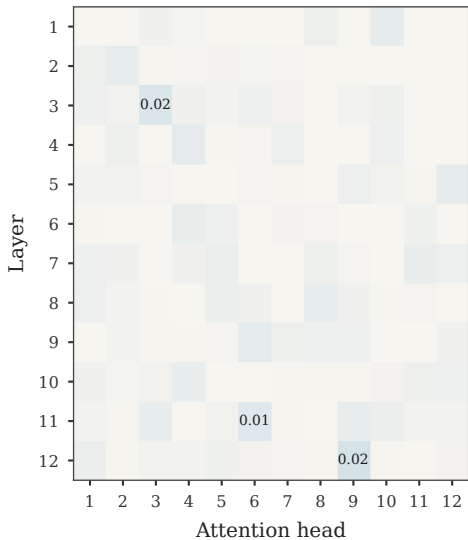
Base GPT-2
